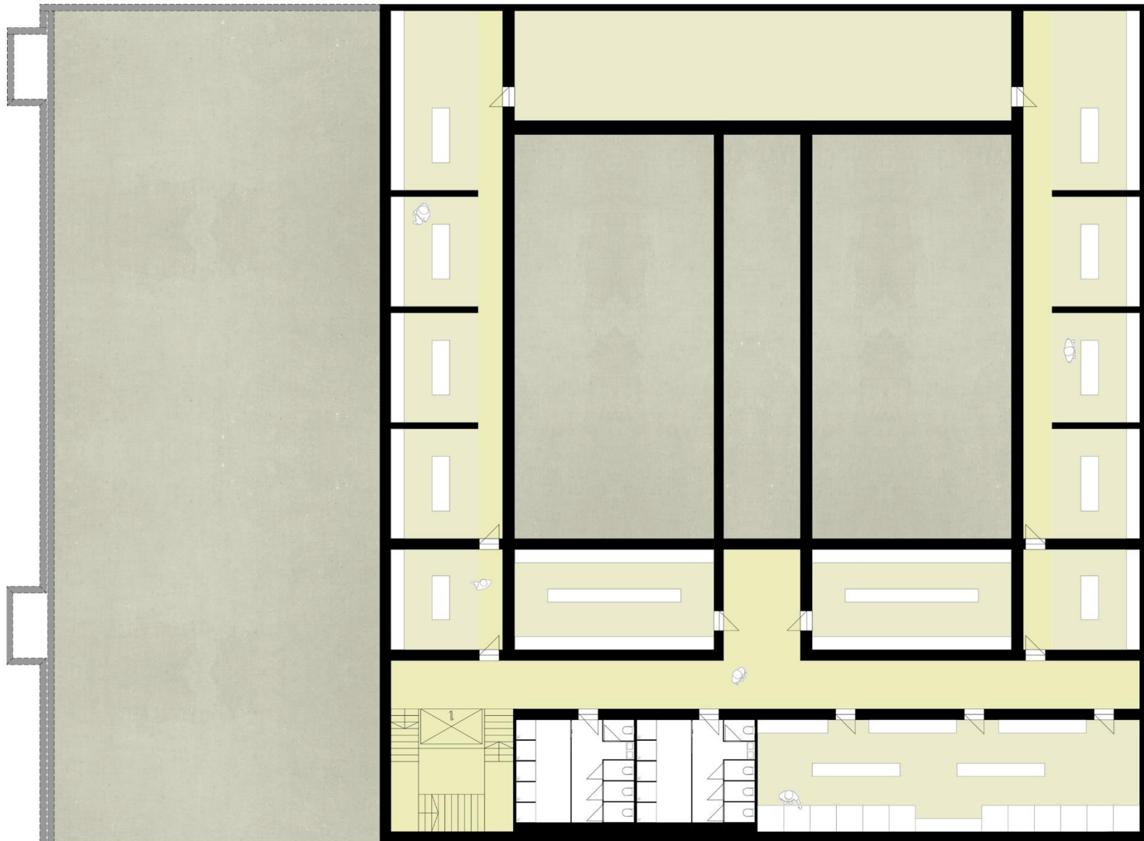
PINCE SZINTI ALAPRAJZ
