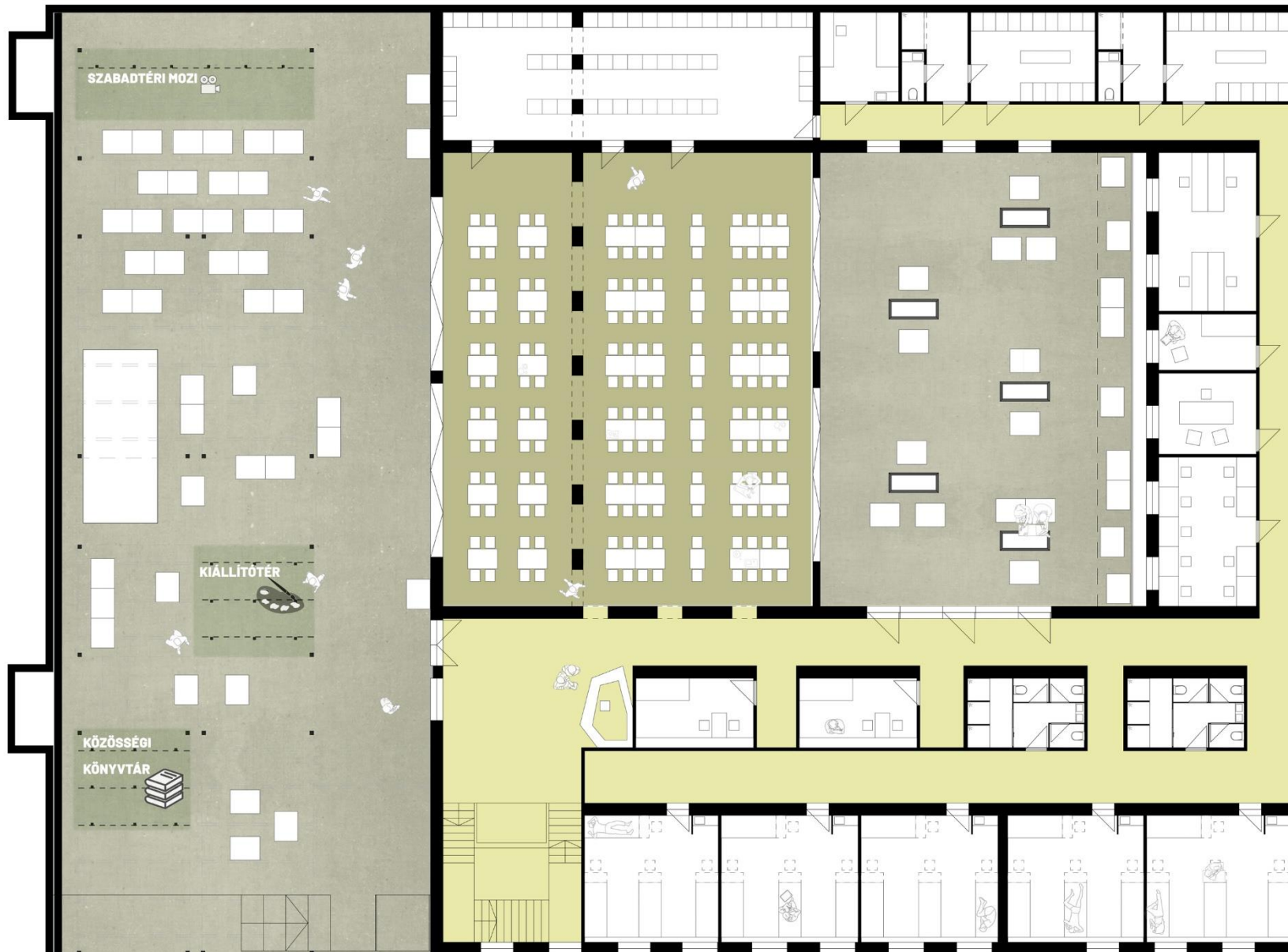
FÖLDSZINTI ALAPRAJZ
