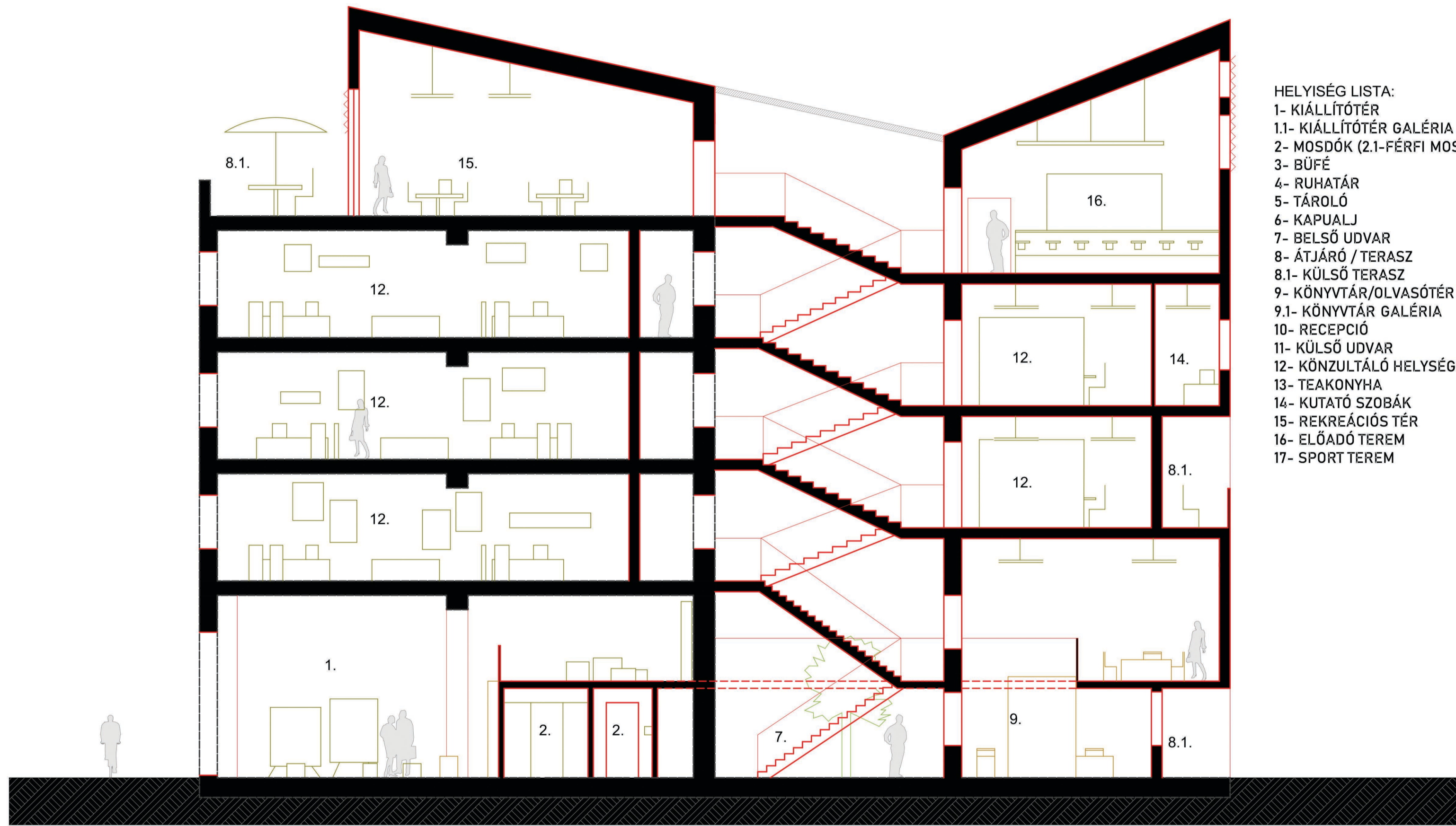
METSZET M 1:100
