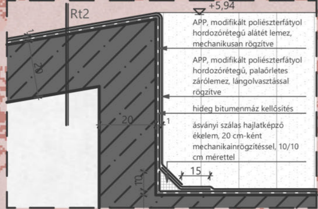
R2 RÉSZLETRAJZ M 1:20
