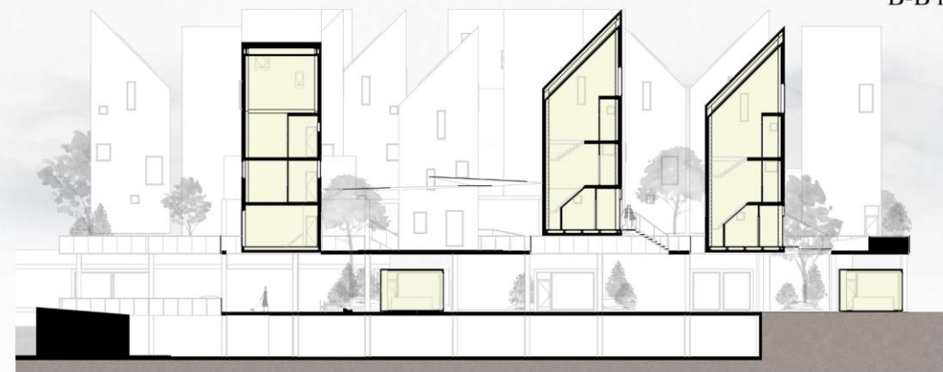
B-B metszet
