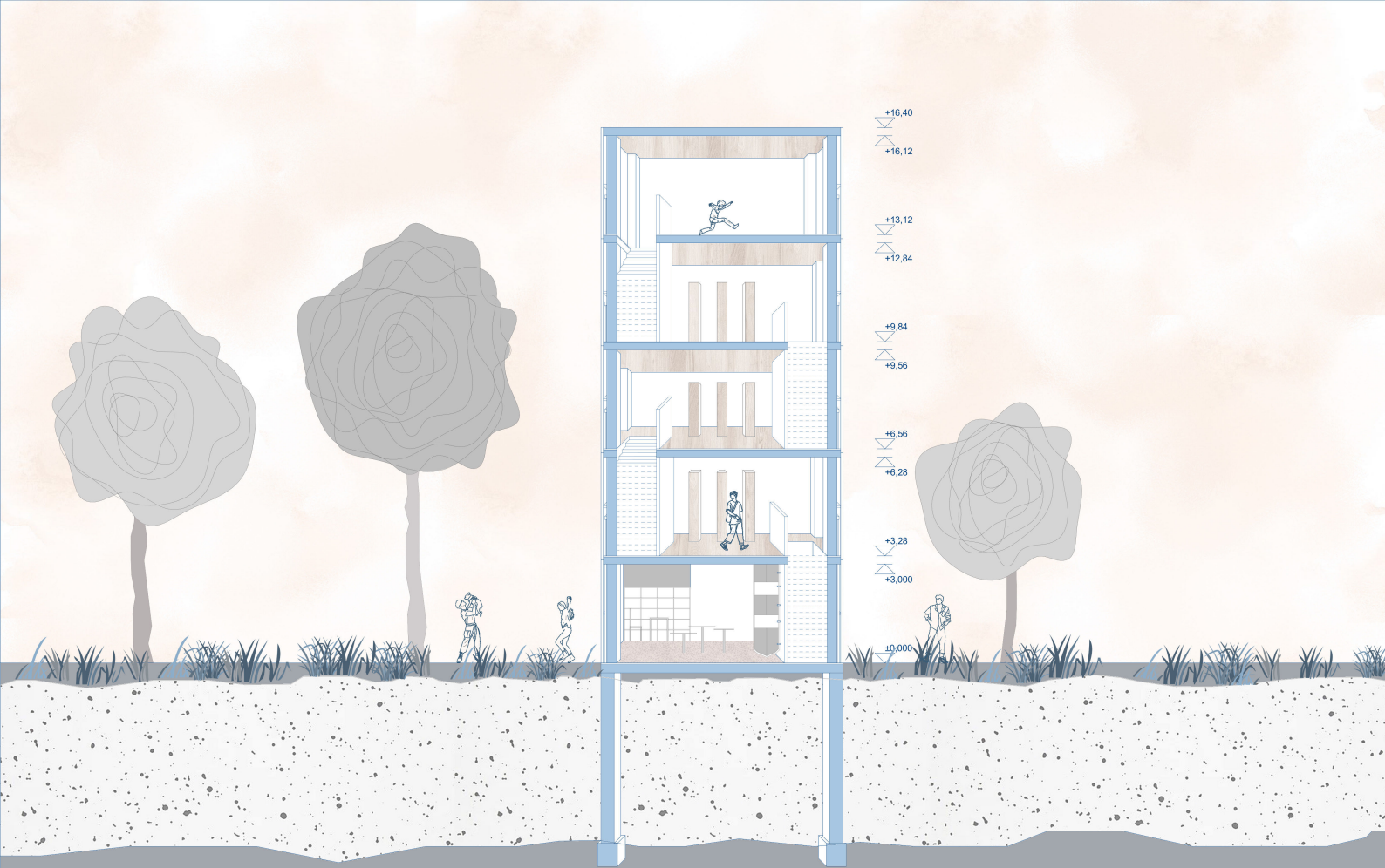
A-A Metszet M=1:100
