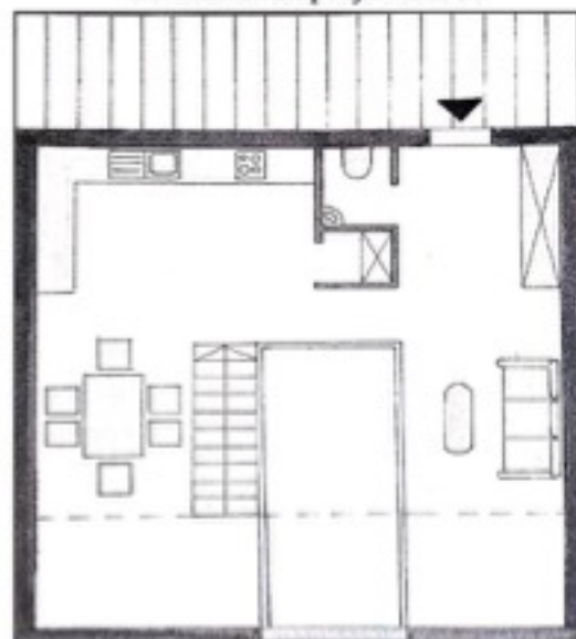
Földszinti alaprajz M1:100
