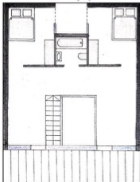
Emeleti alaprajz M1:100
