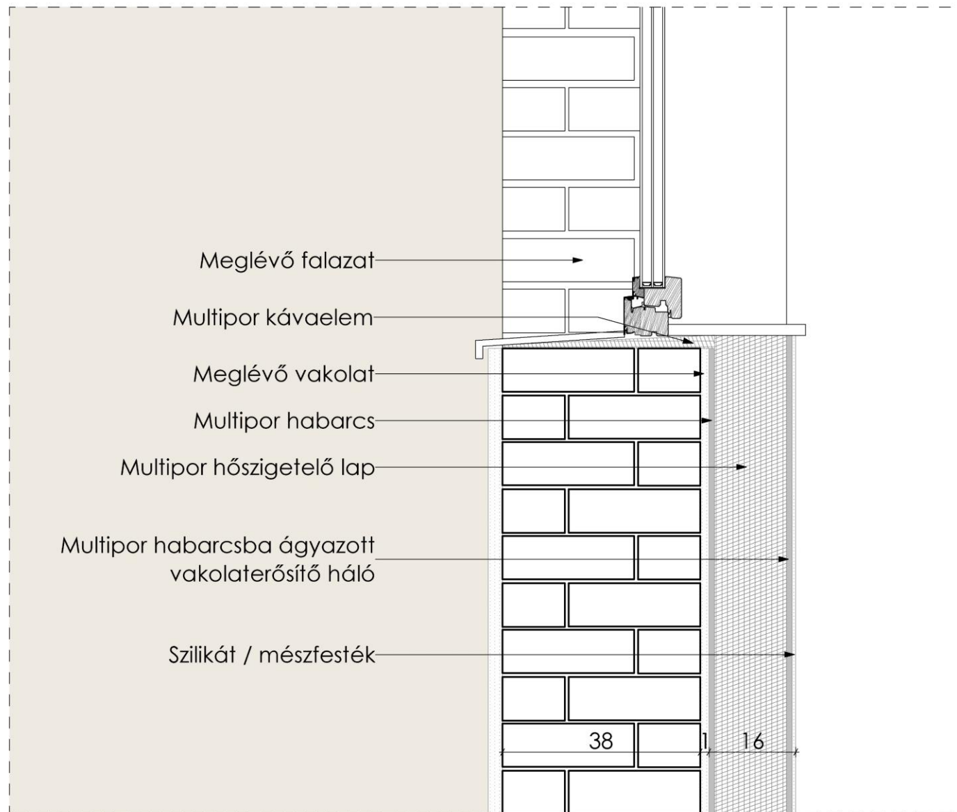
RÉSZLETKÉPZÉS MEGLÉVŐ ÉPÜLET TERMIKUS LEVÁLASZTÁSÁNÁL
