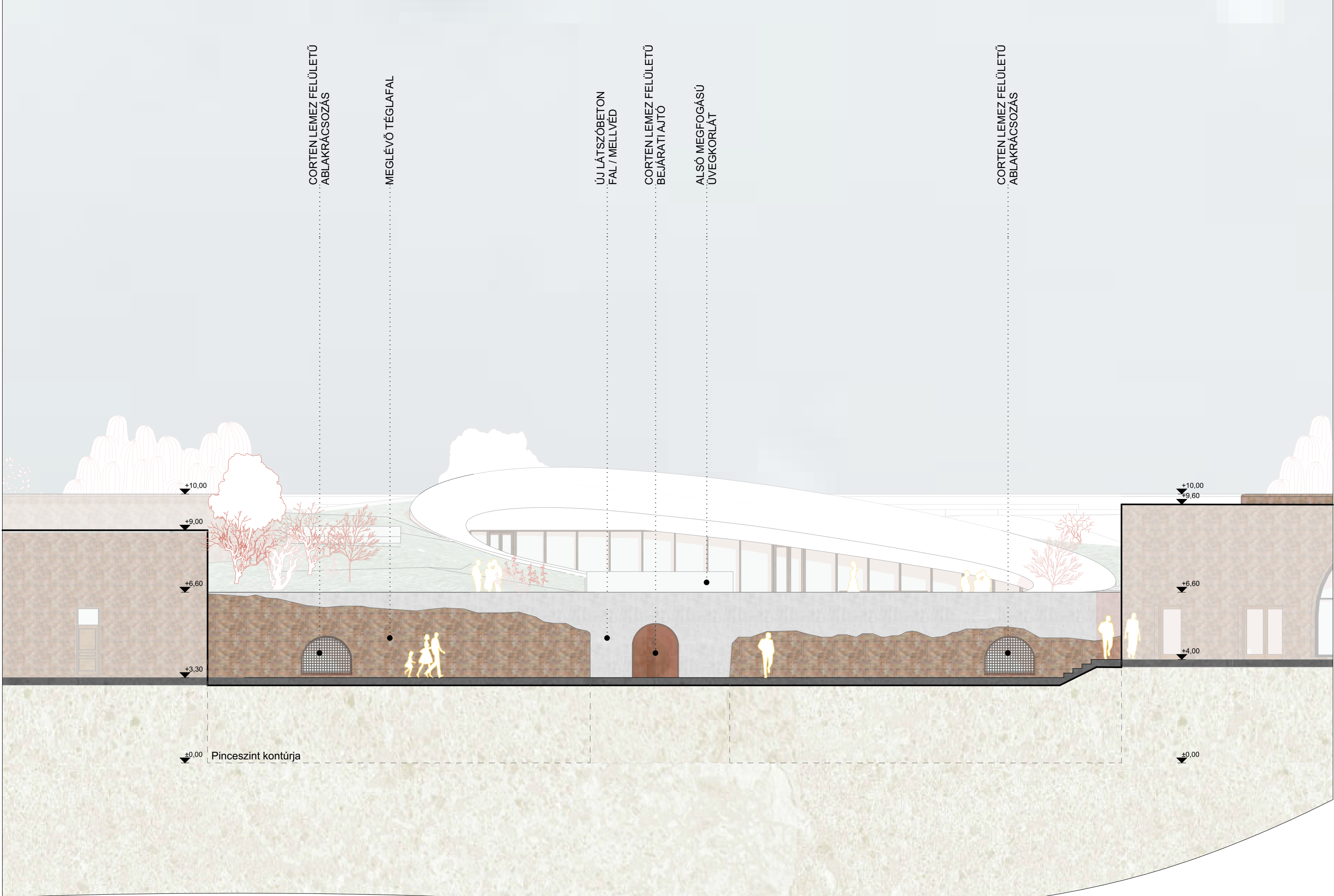
DÉLI HOMLOKZAT - M 1:100
