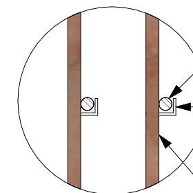
Részletrajz - függőleges metszet M 1:2 két panel csatlakozásánál lévő acél kampó
