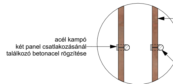
Részletrajz - vízszintes metszet M 1:2
