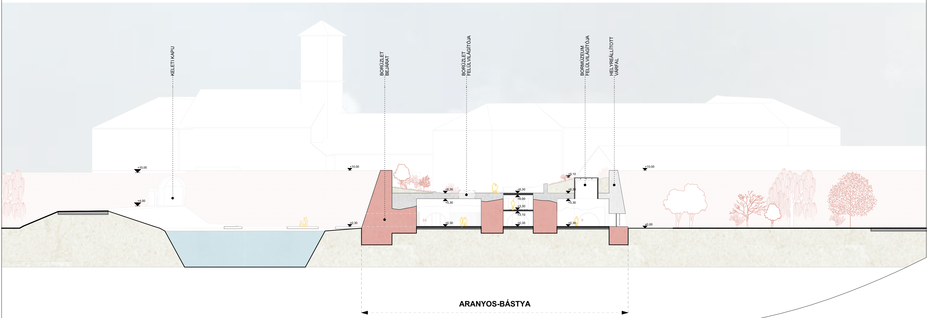
TEREPMETSZETEK - M 1:200
