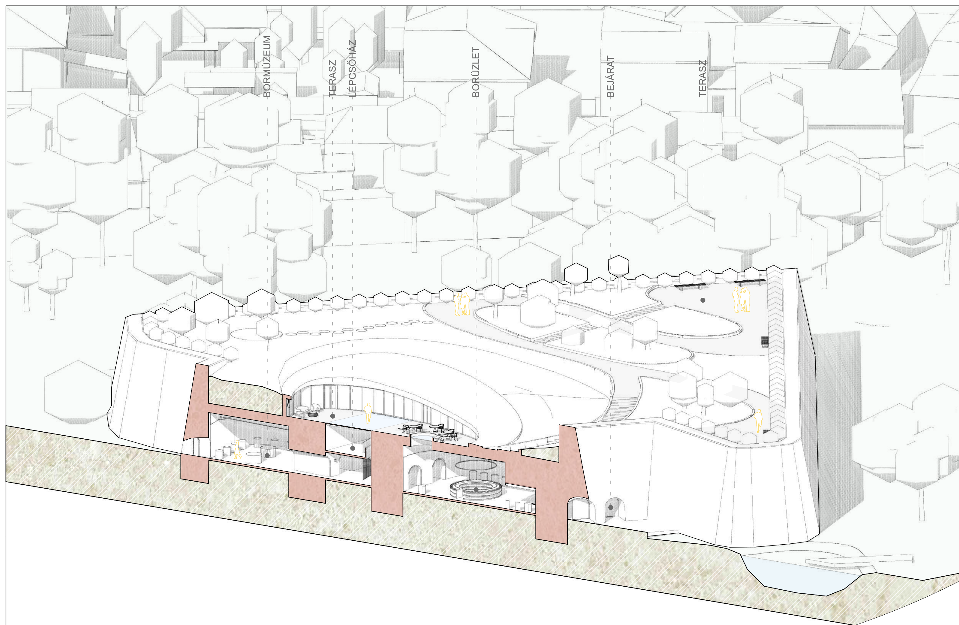
AXONOMETRIA - B-B METSZET
