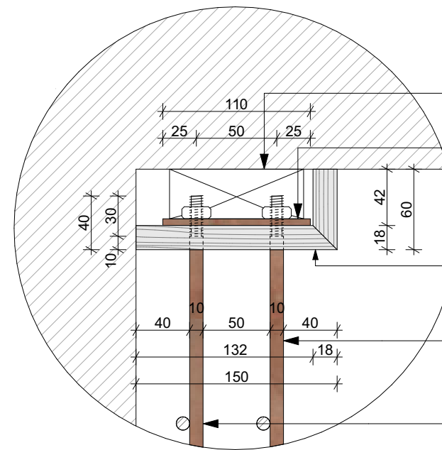
Részletrajz - függőleges metszet M 1:2
