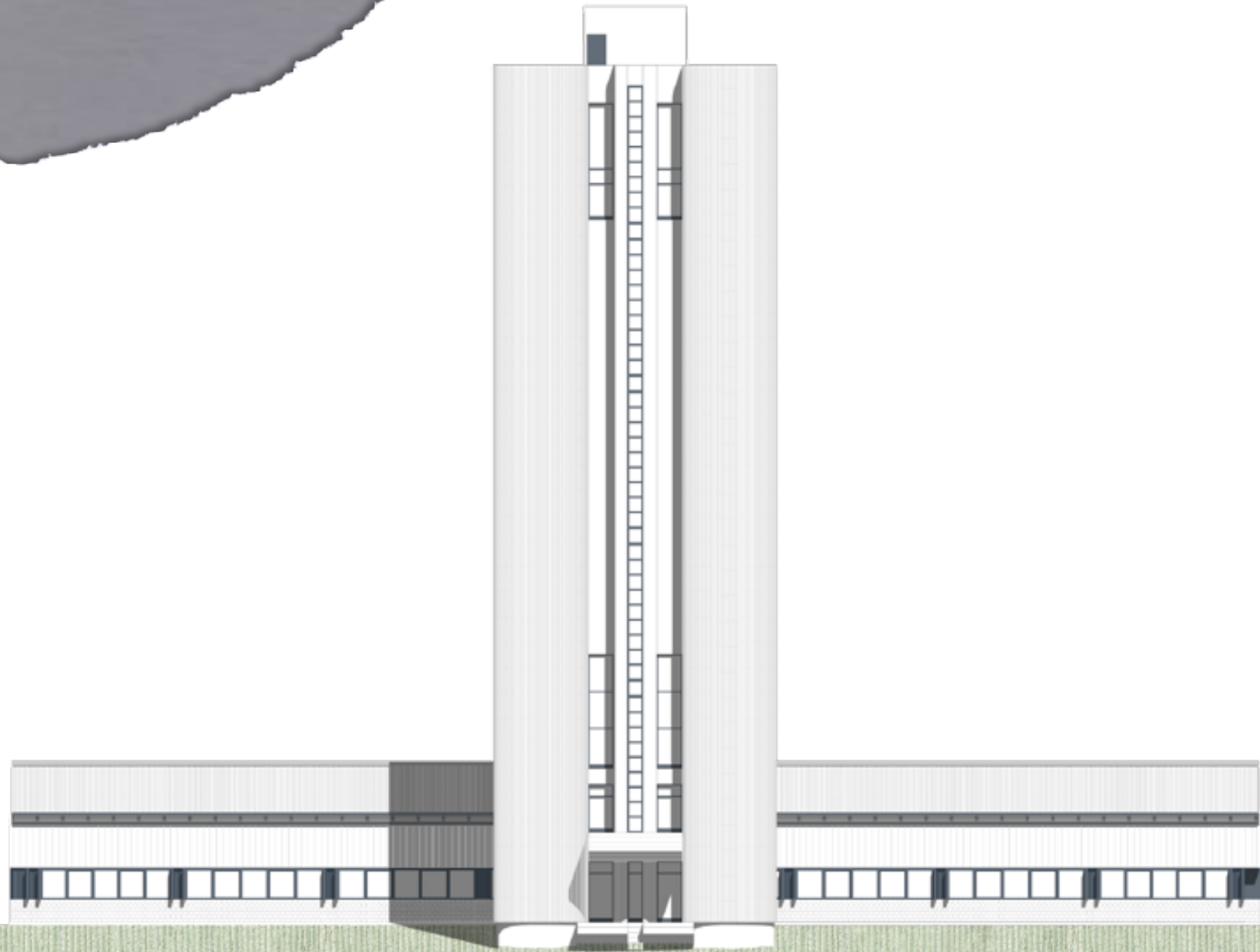
KELETI HOMLOKZAT – MEGLÉVŐ m = 1:200
