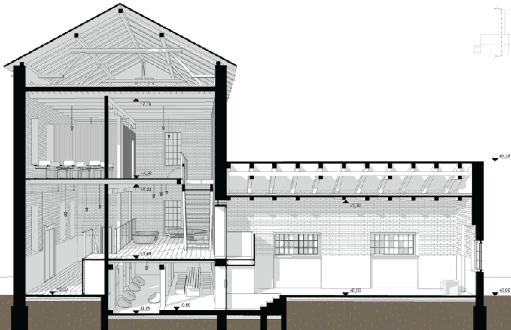
Malom Új B-B metszet
