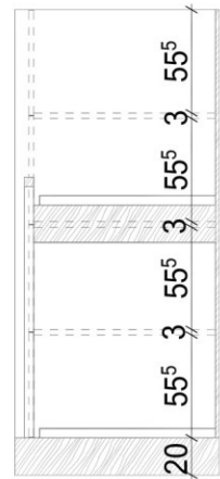
METSZET RAJZ
