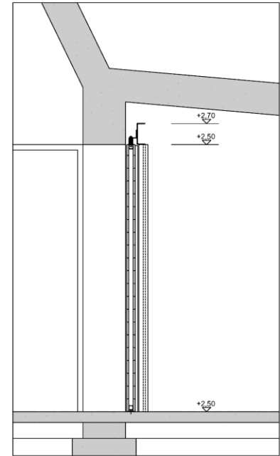
K4 METSZET (TOLÓKAPU-BEJÁRAT)
