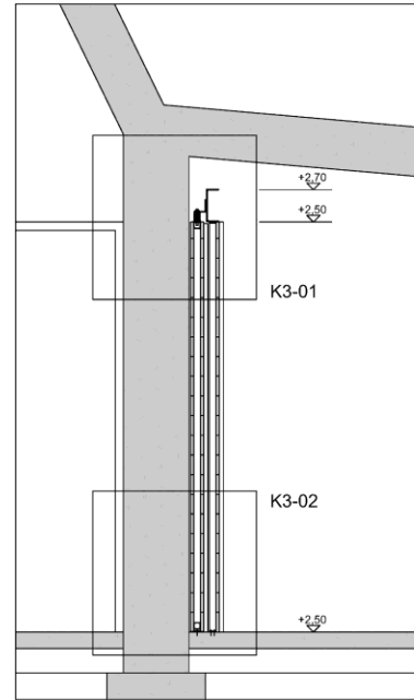
K3 METSZET (TOLÓKAPU)
