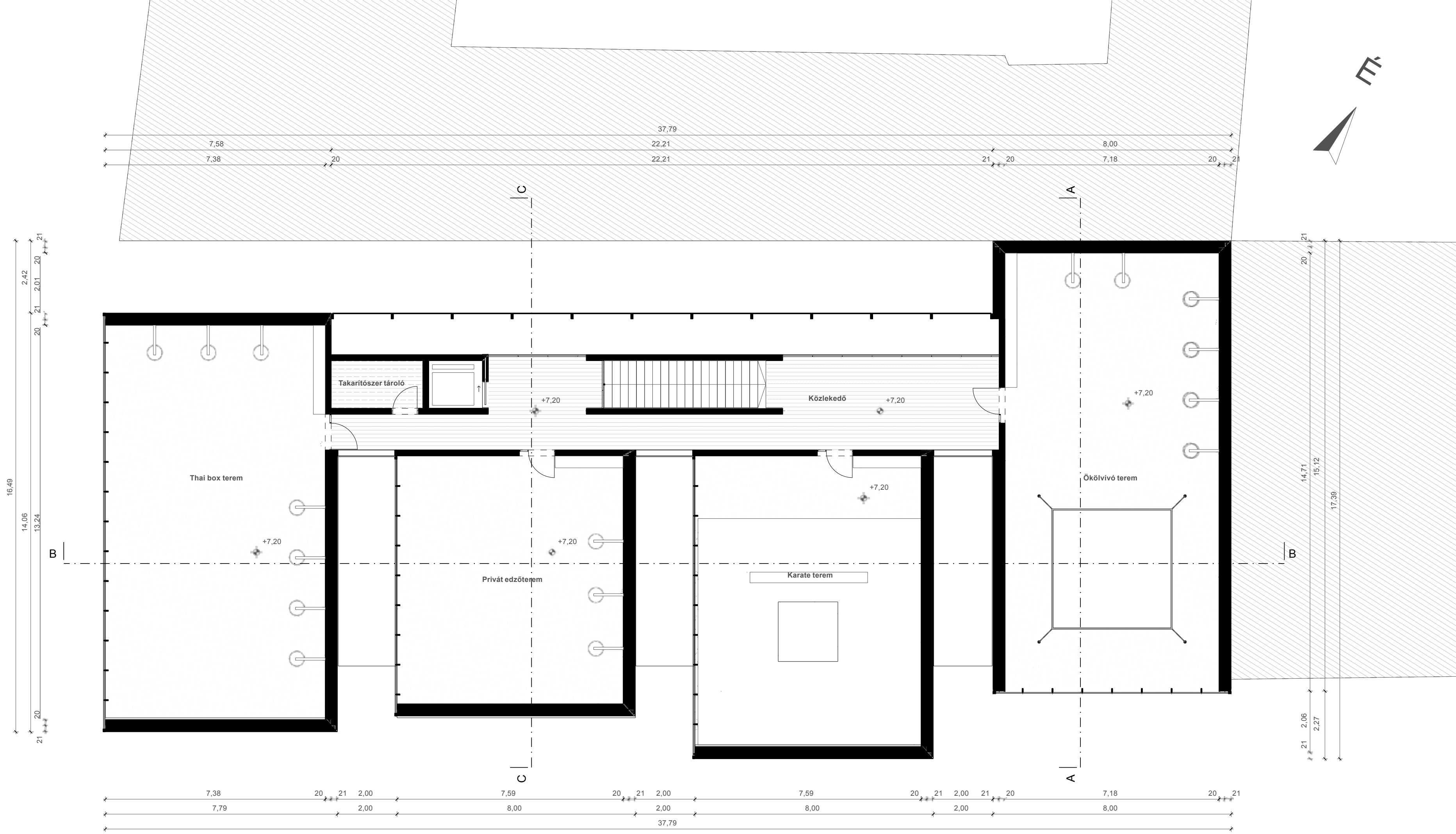
2. EMELETI ALAPRAJZ
