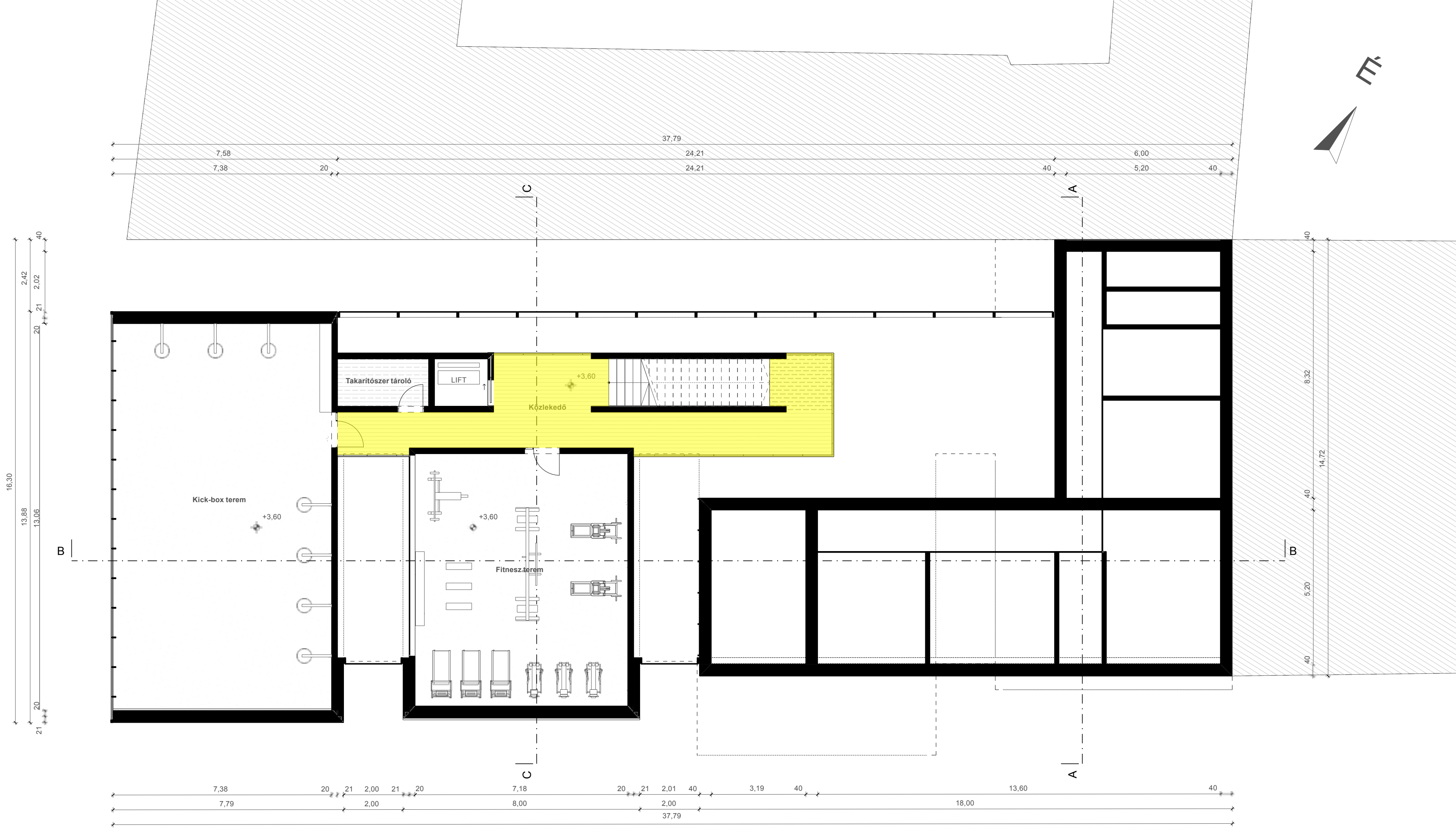
1. EMELETI ALAPRAJZ
