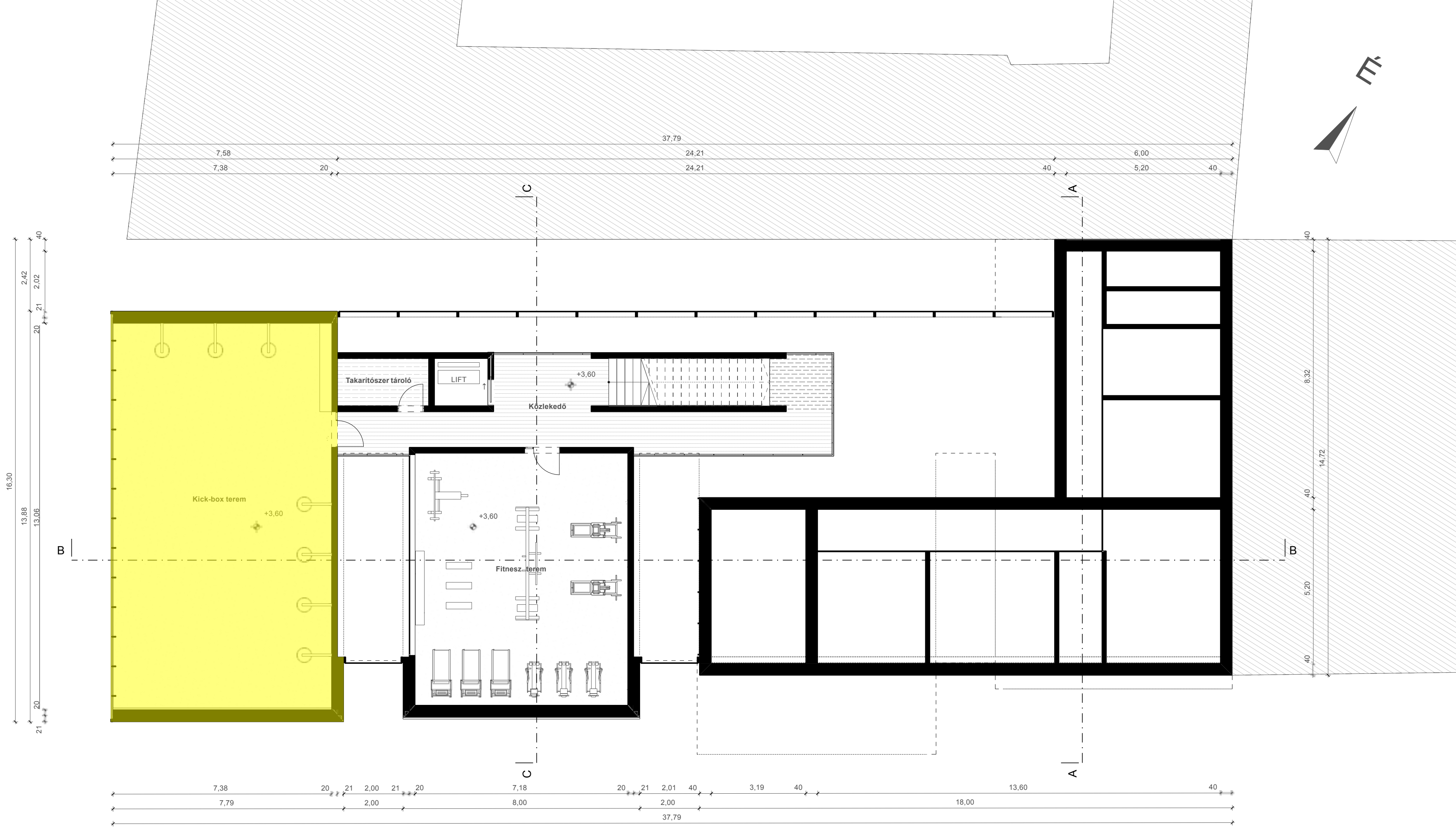
1. EMELETI ALAPRAJZ
