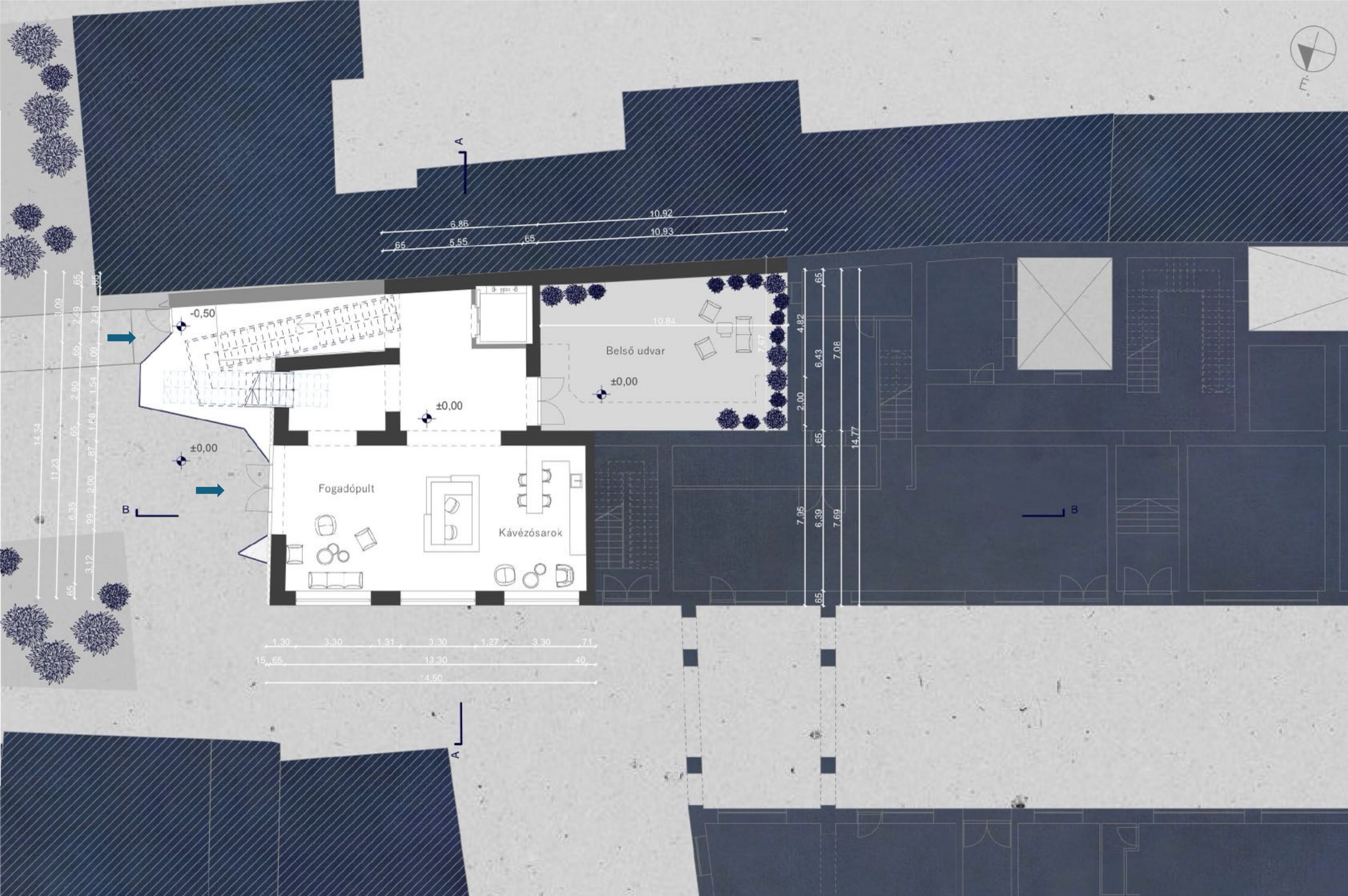
Földszinti alaprajz
