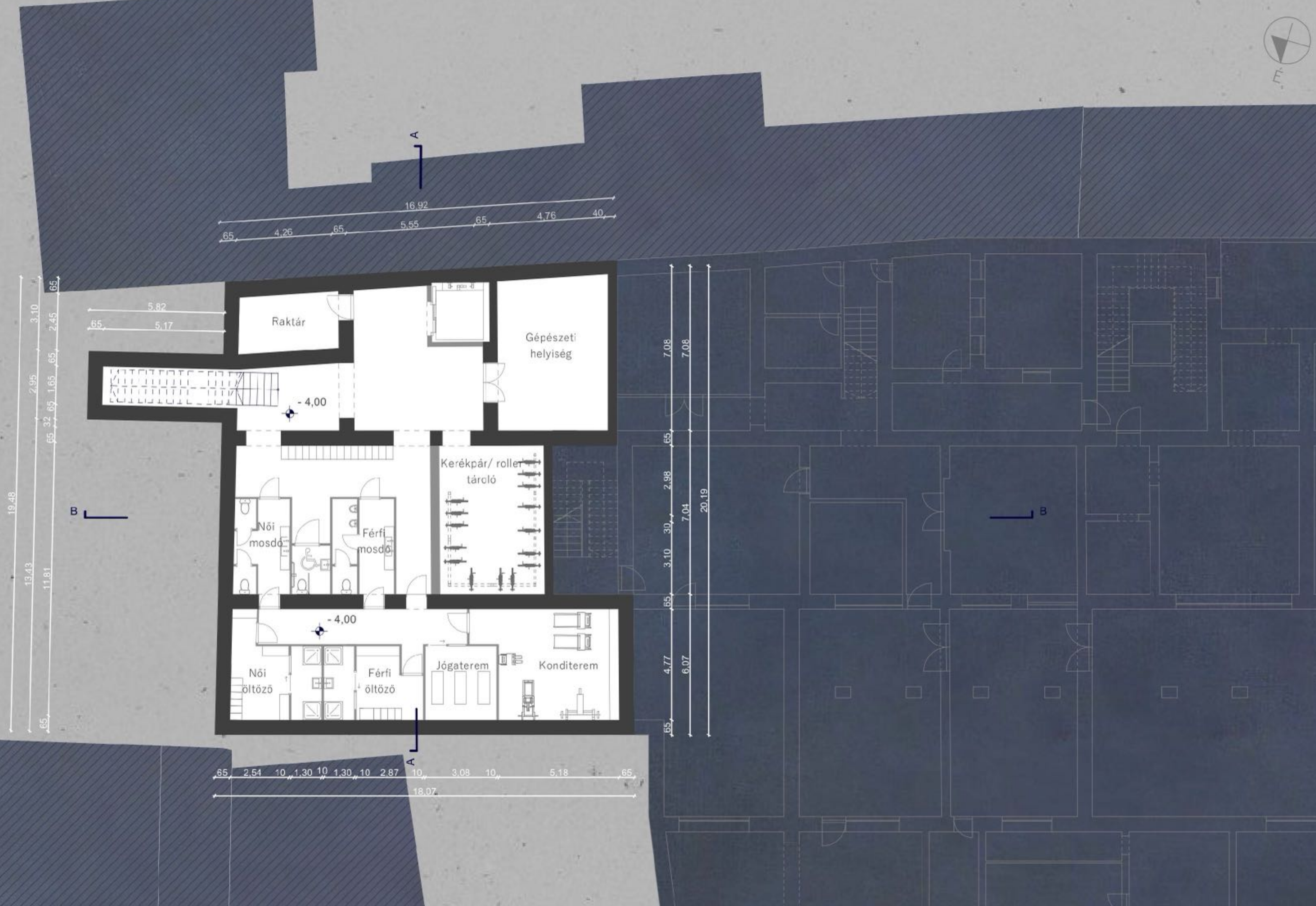
Alagsori alaprajz
