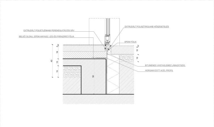
M 1:10
